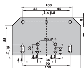
Bevestigingsplaat voor 1600 haak op branddeuren artikelnr. 205231XL
