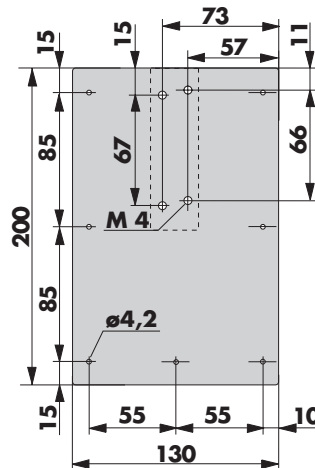
Bevestigingsplaat voor 1600 haak op branddeuren artikelnr. 205231XL
