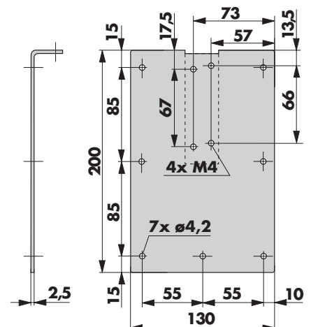
Bevestigingsplaat 1600 voor branddeuren zonder sponning artikelnr. 205237
