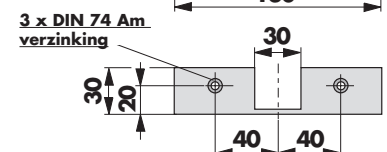
Bevestigingsplaat voor 1600 haak op branddeuren artikelnr. 205231XL
